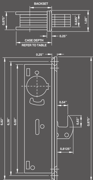
HOOKBOLT
